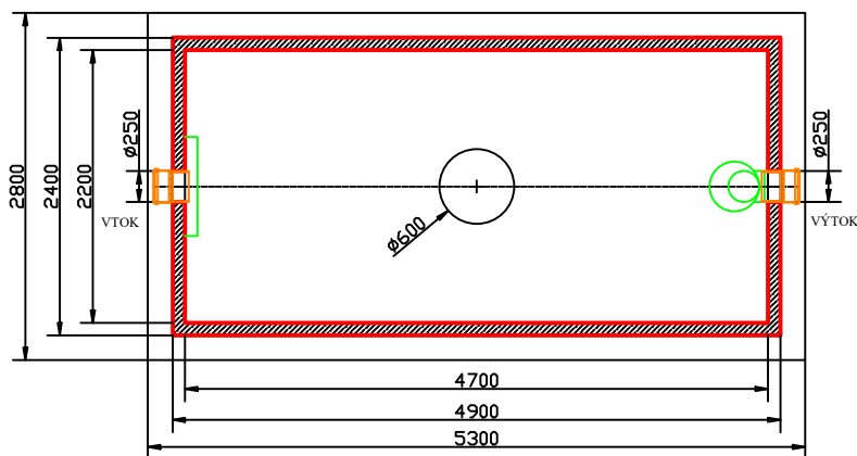
DIMENZIJE OSNOVE PLOČE
