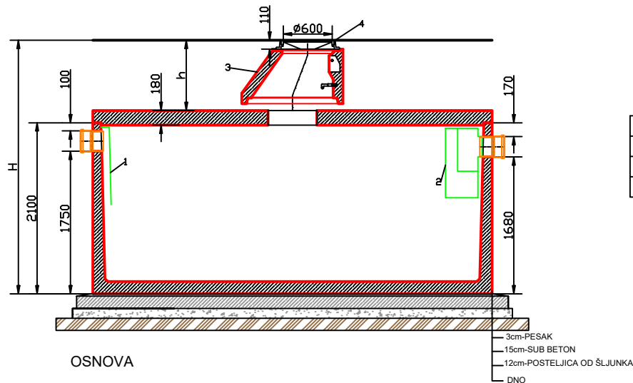
PRESEK A-A'
