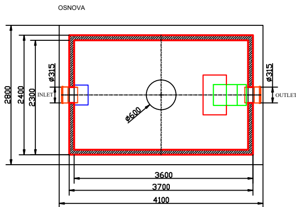
DIMENZIJE OSNOVE PLOČE
