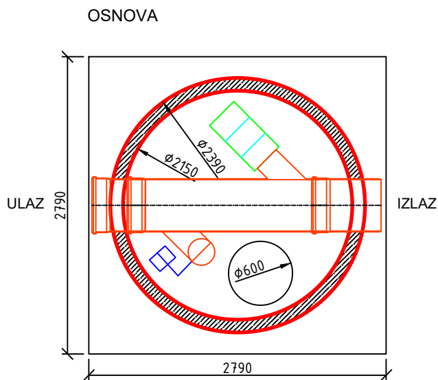
DIMENZIJE OSNOVE PLOČE
