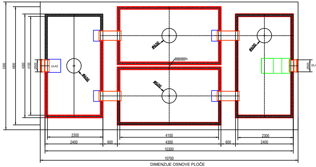
DIMENZIJE OSNOVE PLOČE
