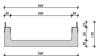
ivica od pocinkovanog čelika CH 120 mm
