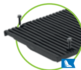
Liveno gvozdena dizajn rešetka KIARO, klasa D, SW 7 šrafljenje sa 4 šrafa
