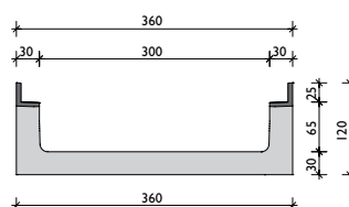
Liveno gvozdena ivica CH 120 mm
