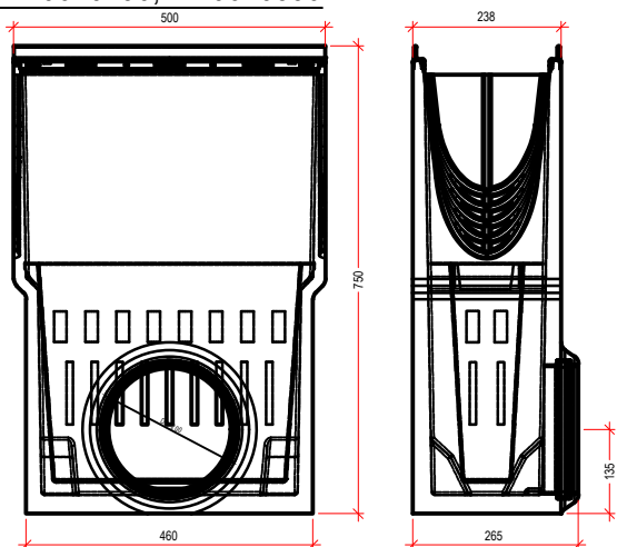
Kanal - dimenzije
