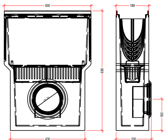
Kanal - dimenzije
