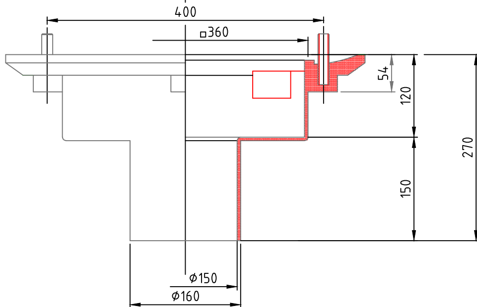
Presek A-A
