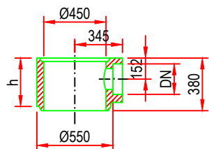
Izliv za betonsku cev, bez sifona 5003-DN 150 5003-DN 200
