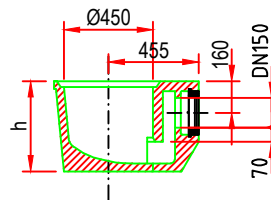
Izliv za betonsku cev, sa sifonom DN 150 5001-150MGV-L
