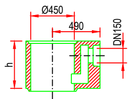
Izliv za betonsku cev DN150, sa sifonom 5003-150MGV
