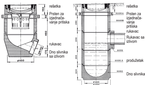
Prsten za izjednačavanje pritiska sa držačem za koficu
